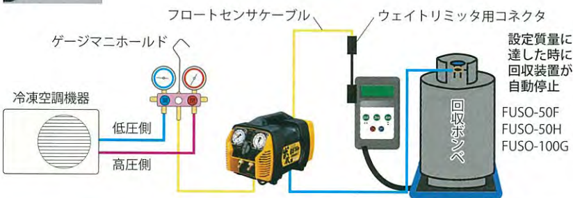
ウェイトリミッターコネクタ取付図
